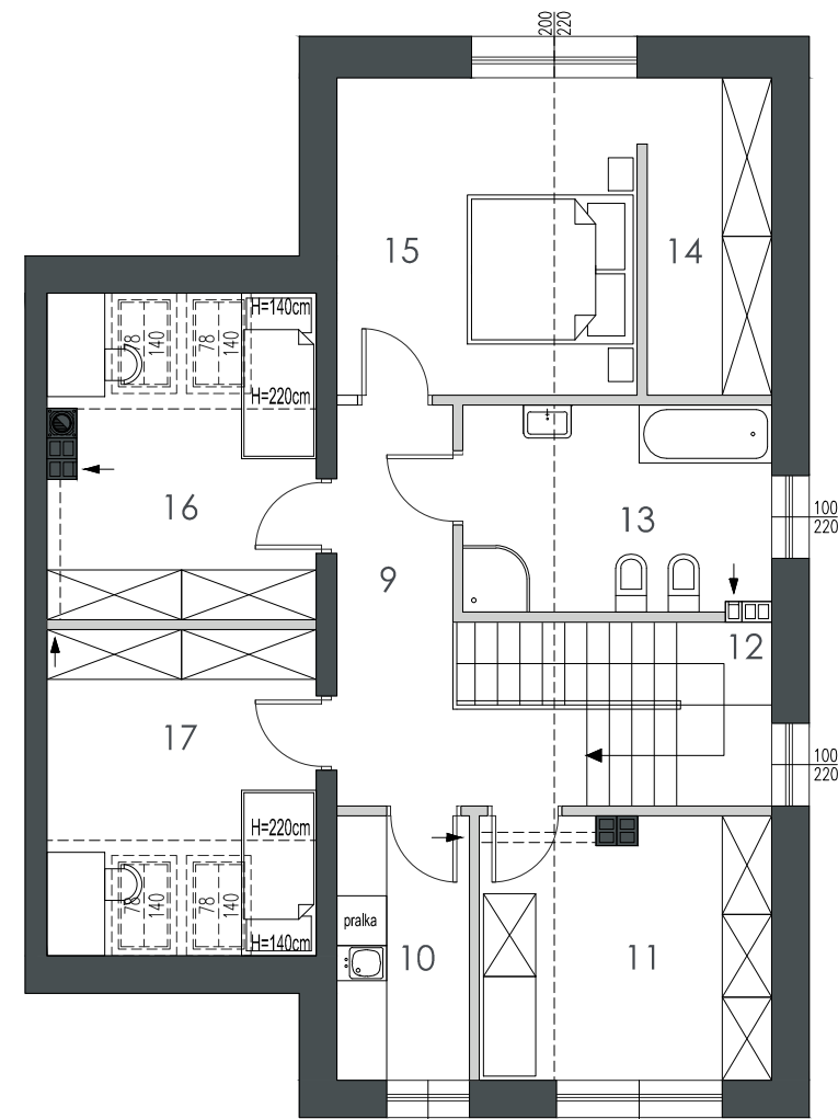
rzut poddasza
